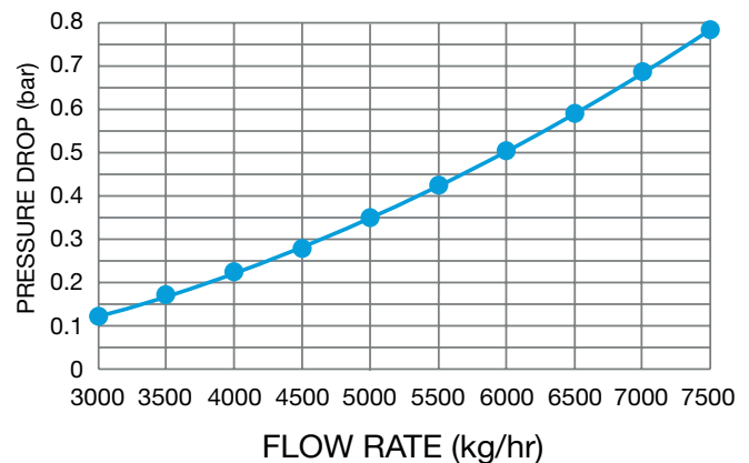
CV15: Pressure Drop v Flow At -163°C LNG
