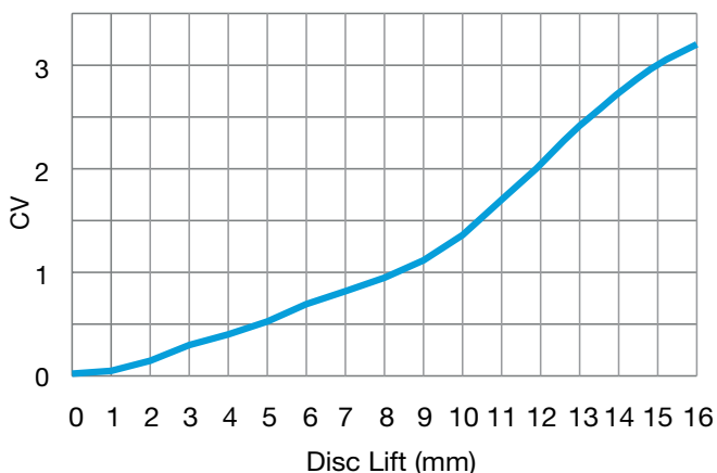
CV vs Disc Lift at -165°C LNG
